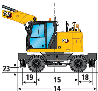
Laufwerk mit 2 Sätzen Abstützpratzen
