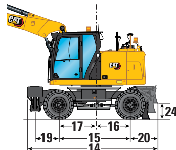
Laufwerk mit 1 Paar Abstützpratzen und Schild
